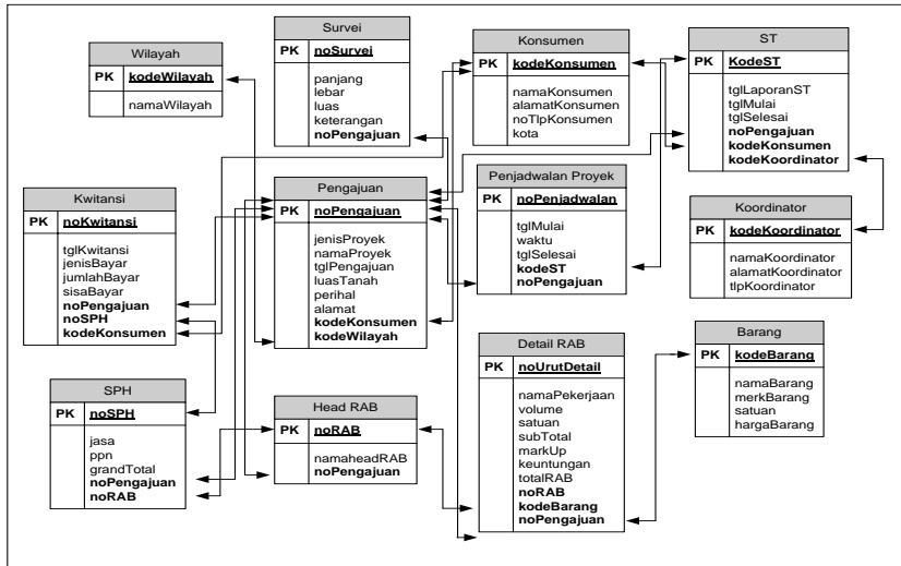
Gambar 4. Tabel Relasi
